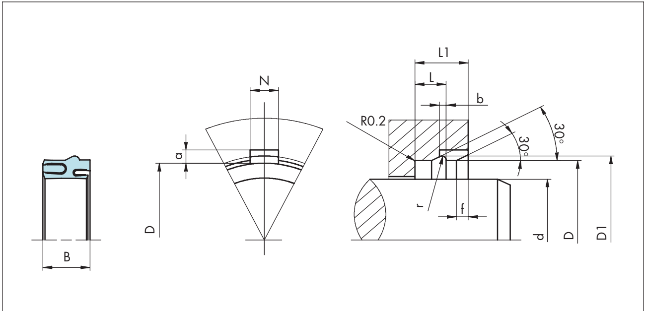
图16 安装图
