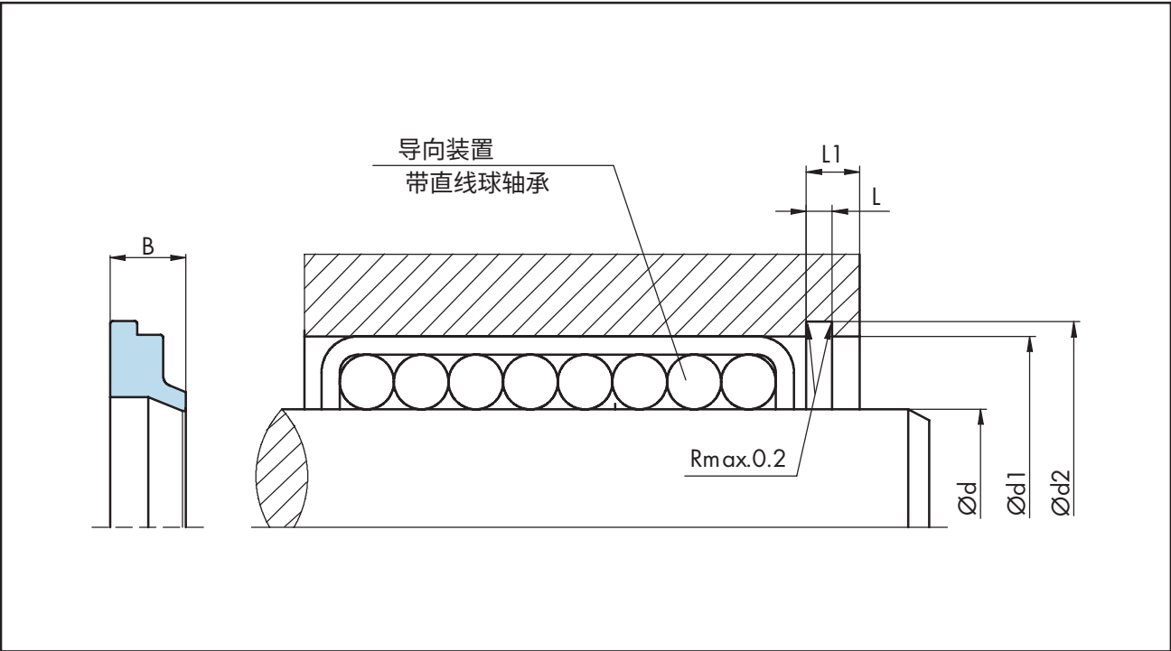
图15 安装图
