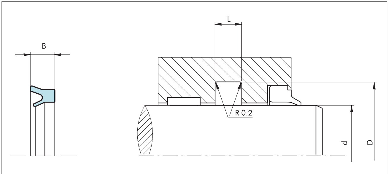
图3 安装图
