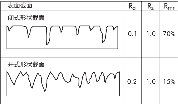
图2 表面的形状截面
