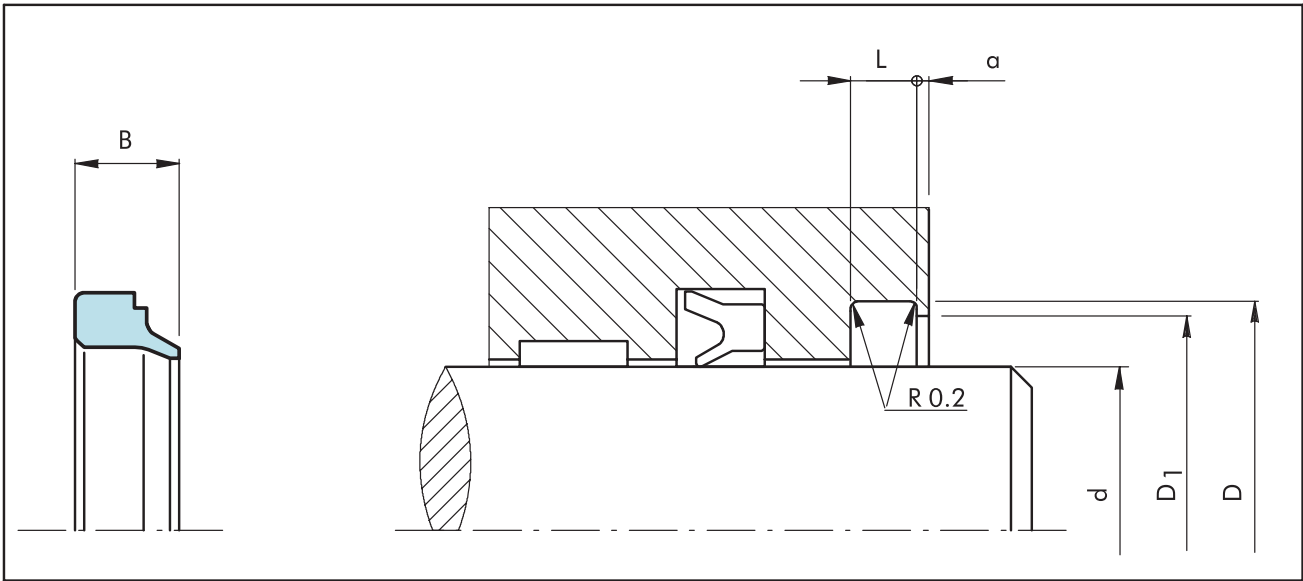
图14 安装图
