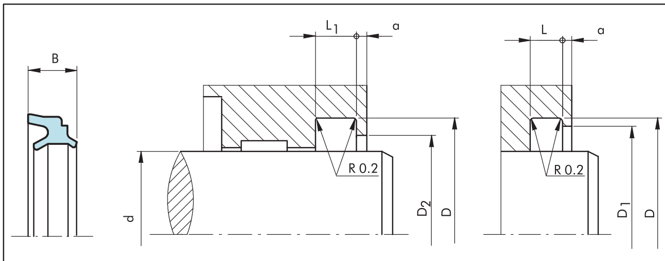
图12 安装图
