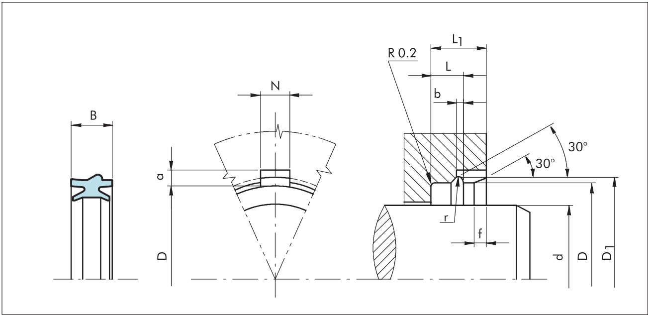
图13 安装图
