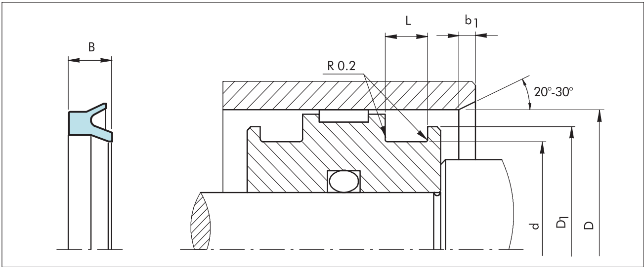
图5 安装图
