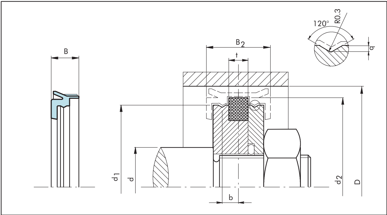
图7 安装图
