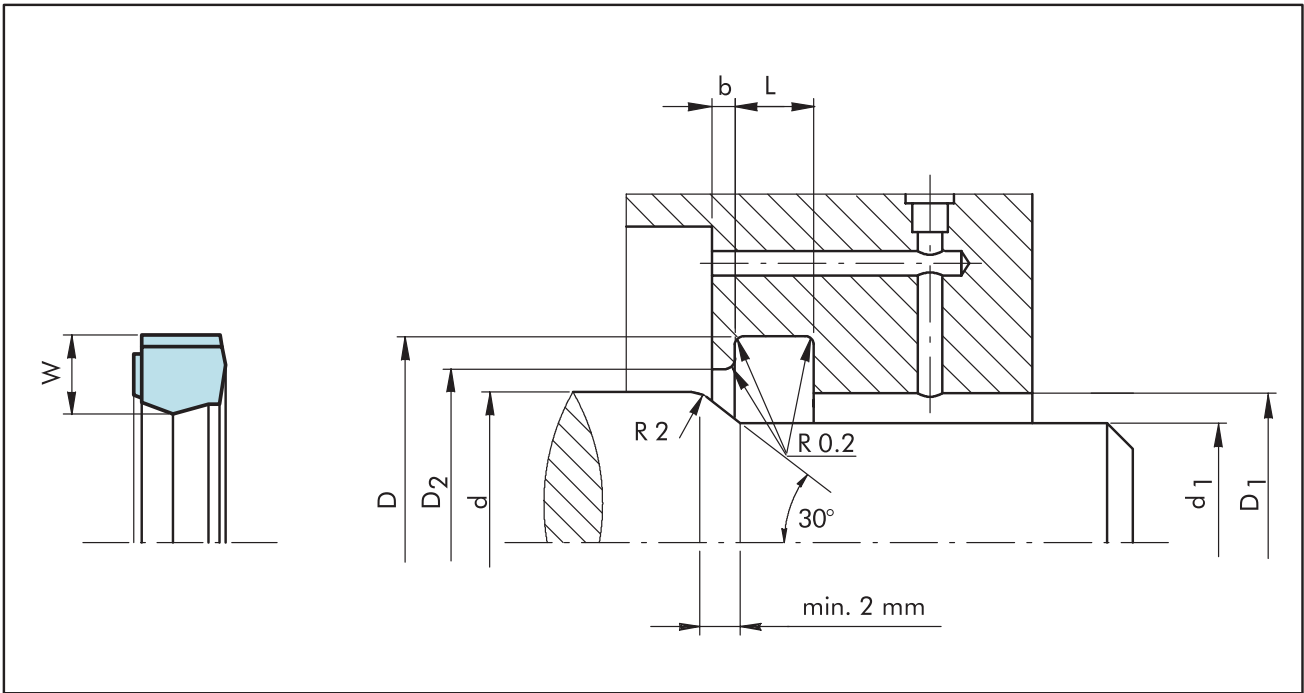
图18 安装图
