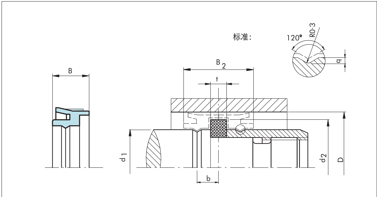
图6 安装图
