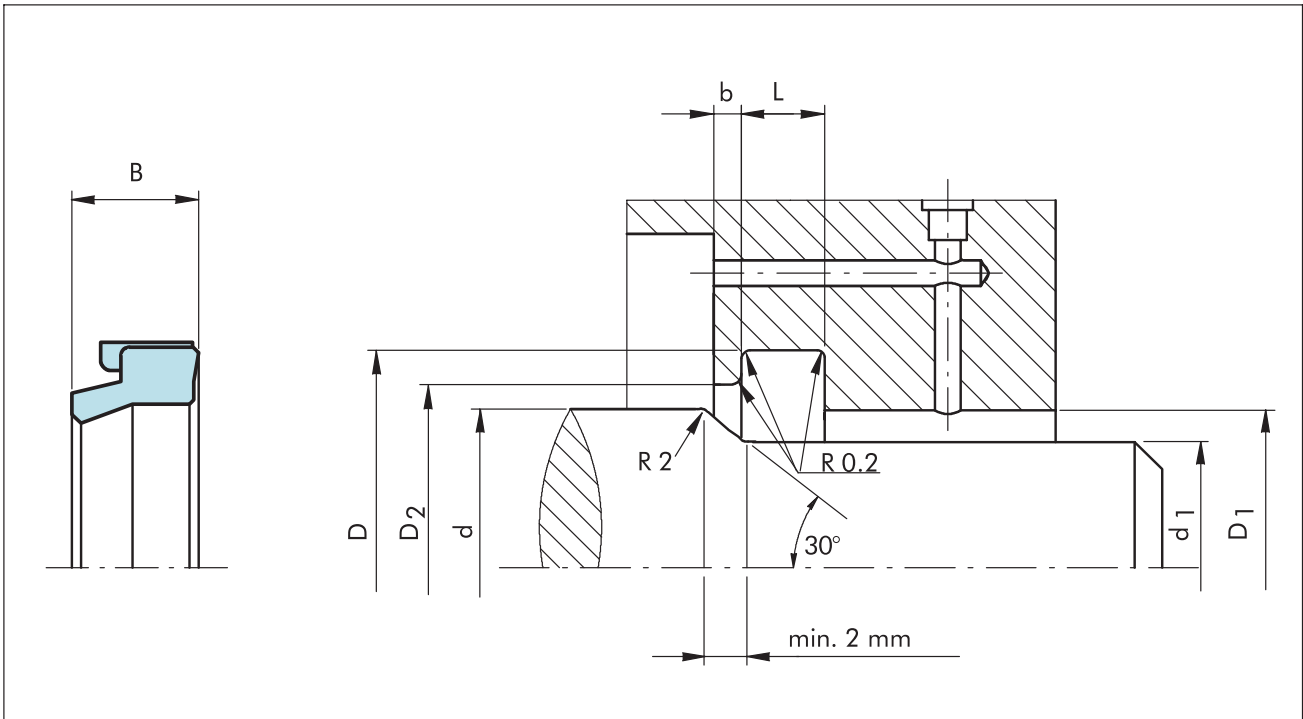
图17 安装图
