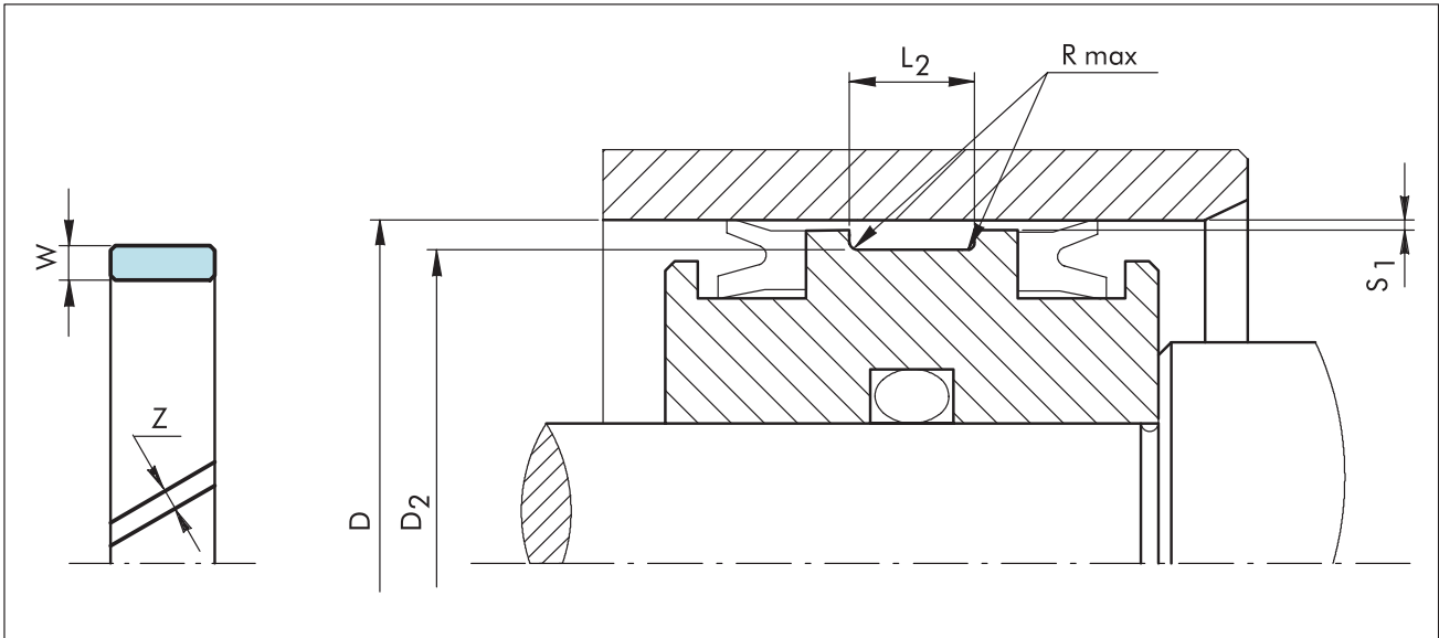
图19 安装图
